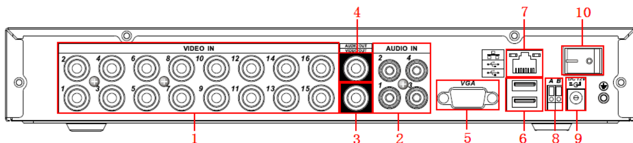
Rysunek 2-2c. Wygląd tylnego panelu rejestratora 16-kanalowego.
