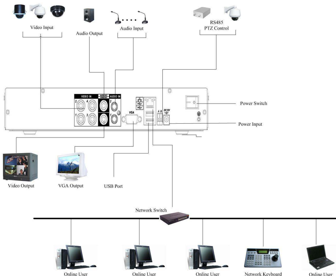
Rysunek 2-5a. Przykładowy schemat podłączenia urządzeń peryferyjnych do rejestratora 8-kanalowego serii LE-A.
