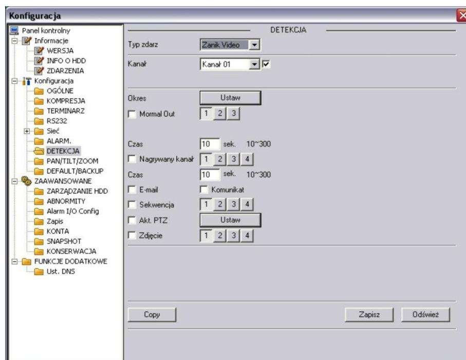
Rys. 7-42. Panel kontrolny → Konfiguracja → Detekcja → Zanik Video.
