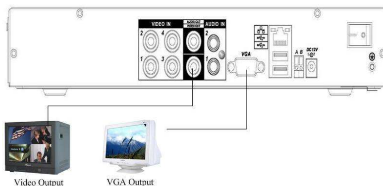
Rys. 3-2. Podłączenie monitorów do rejestratora
