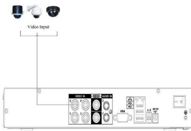
Rys. 3-1. Przykładowe podłączenie kamer do rejestratora
