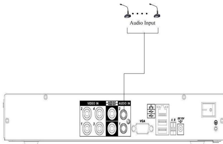
Rys. 3-3. Podłączenia wejść i wyjść audio do rejestratora 4-kanalowego.
