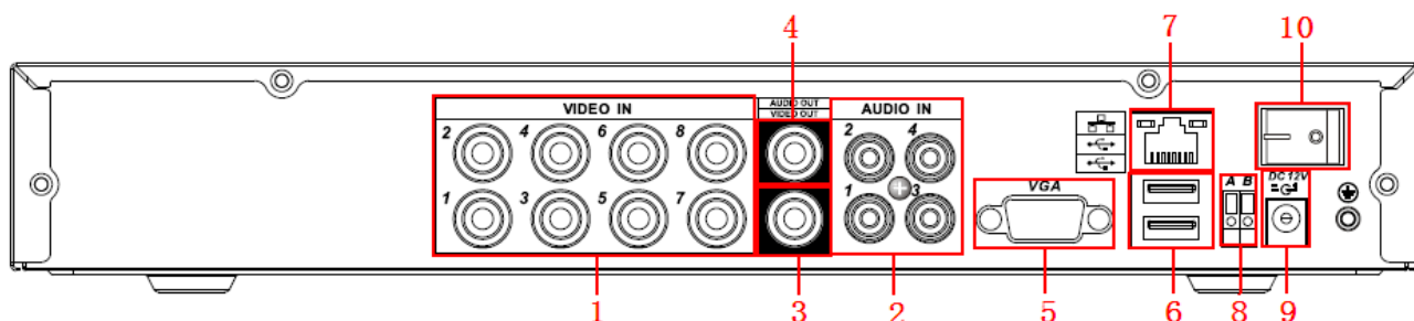
Rysunek 2-2b. Wygląd tylnego panelu rejestratora 8-kanalowego.
