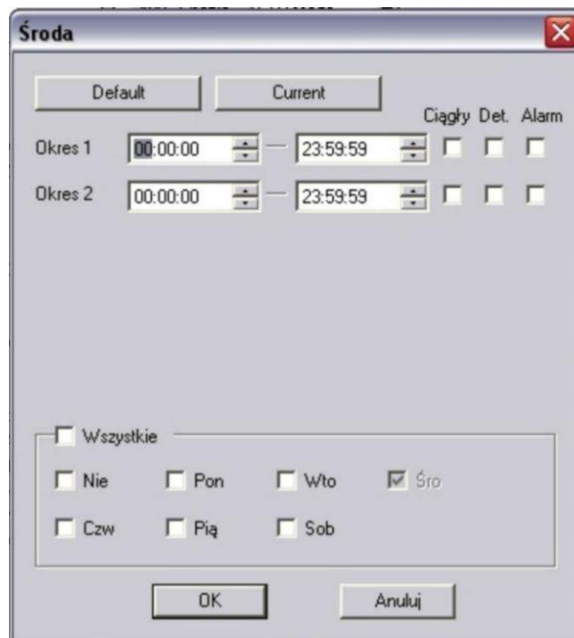
Rys. 7-36a. Interfejs ustawiania terminarza dla funkcji FTP
