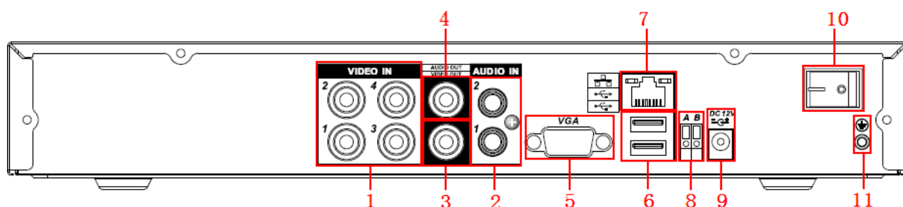
Rysunek 2-2a. Wygląd tylnego panelu rejestratora 4-kanalowego
